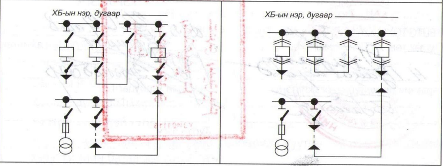
1.3 Компанийн хуваарилах байгууламжаар дамжин тэжээгдэж буй хэрэглэгчийн дэд өртөөг зааглах схем
