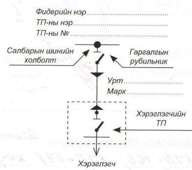
1.3 Компанийн хуваарилах байгууламжаар дамжин тэжээгдэж буй хэрэглэгчийн дэд өртөөг зааглах схем
